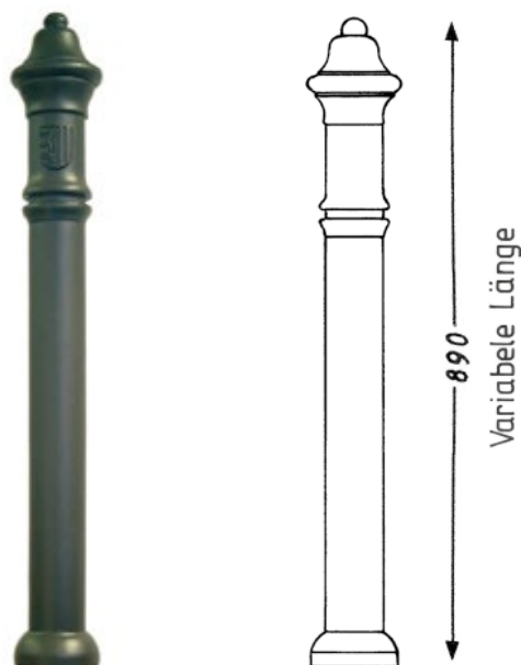
TAP-2008-1 / TAP-2008-2 / TAP-2008-3 Gewicht: ??kg / Bodenhülse aus Stahl Variationen: TGP-2008-y / TAB-2008-y
